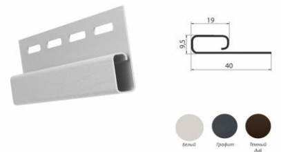
Финишная планка
